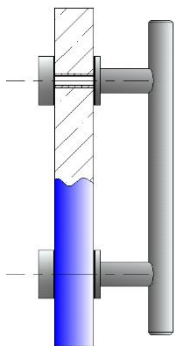
Typ - 02 Glastür als Einzelgriff Einseitige Befestigung Glasbohrung d:14,0 d:14,0 mm +0,5
