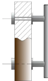
Typ - 04 Holztür # 38-80mm als Einzelgriff Einseitige Befestigung sichtbar Bohrung d:10,0 mm
