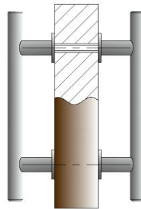
Typ - 03 Holztür # 38-80mm als Griffpaar Bohrung d:10,0 mm
