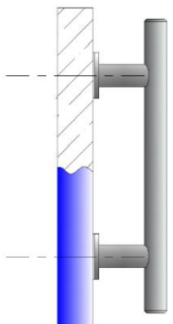
Typ - 07 Glastür UV-Verklebung
