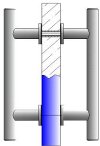
Typ - 01 Glastür als Griffpaar 8-12mm Glasbohrung d:14,0
