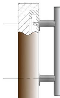
Typ - 06 Aluminiumtür und Profiltür als Einzelgriff Unsichtbare Befestigung mit Einschneideschraube
