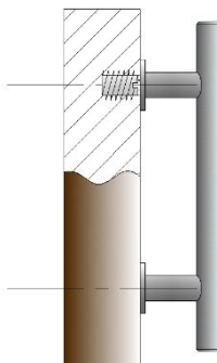
Typ - 05 Holztür und Profiltür als Einzelgriff Unsichtbare Befestigung mit Rampa mufte Bohrung d: 12,0 mm / M8 Gewindestift
